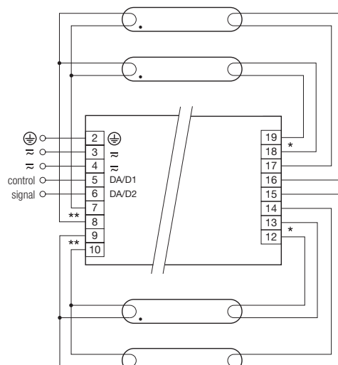
PCA T8 EXCEL one4all Ip xitec 4x18W
