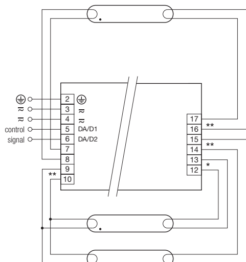
PCA T8 EXCEL one4all Ip xitec 3x18W
